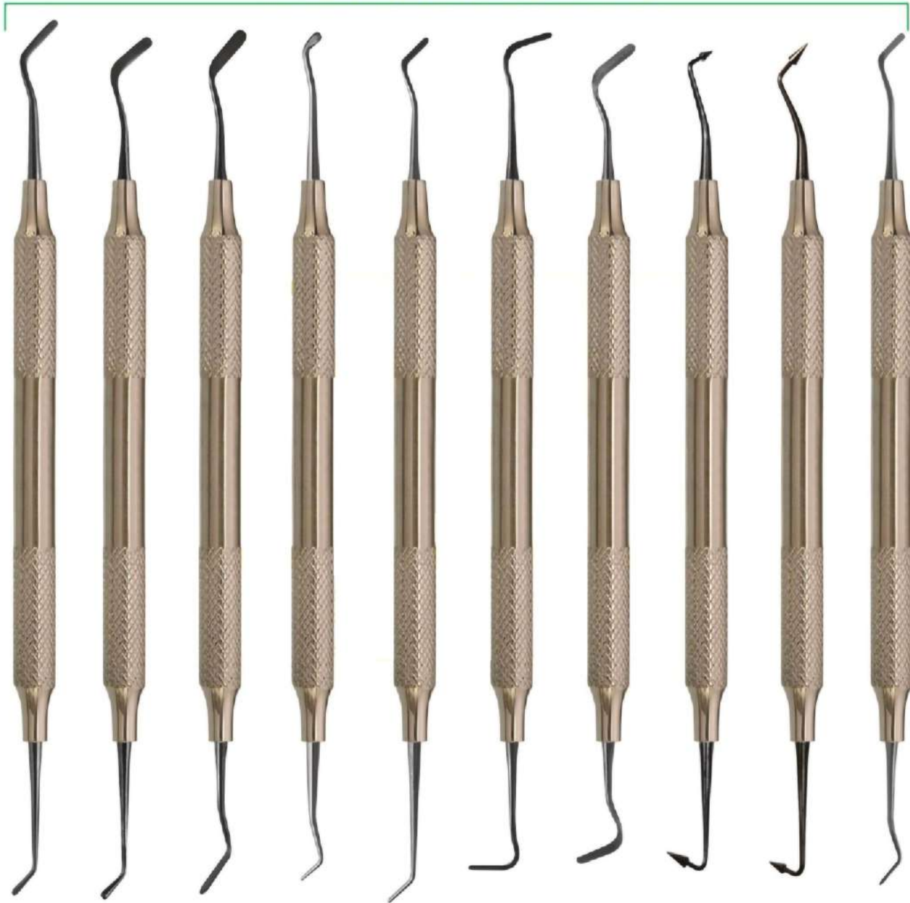
BX-1455 #1 BX-1456 #2 BX-1457 #3 extra flex BX-1458 Micro mini BX-1459 Mini 1 BX-1460 Mini 4 Extra flex BX-1461 # 4 Extra flex BX-1462 #5 flex thin BX-1463 #6 flexi thin BX-1464 Mini 3 Extra flex
